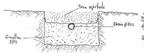
COUPE de PRINCIPLE du lit d'épandage
