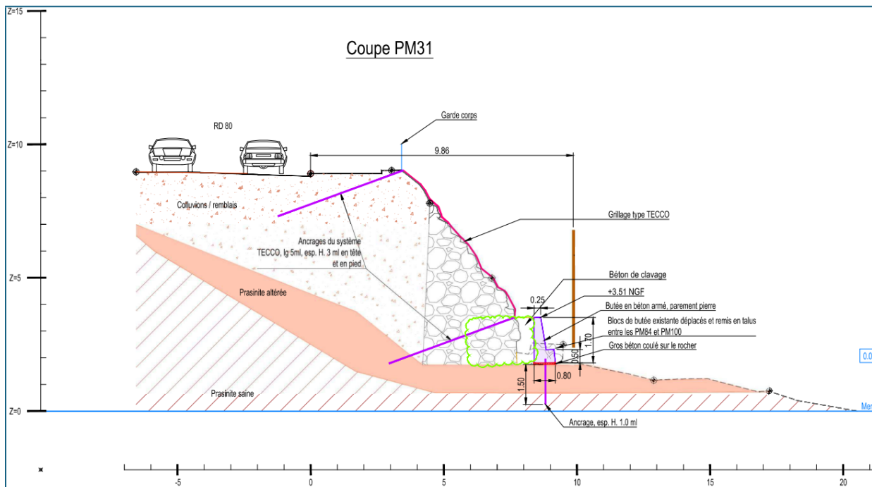
Renforcement du pied de l'ouvrage et confortement du talus en enrochement
