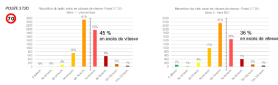
Figure 22 : Répartition des classes de vitesses - Poste 3
